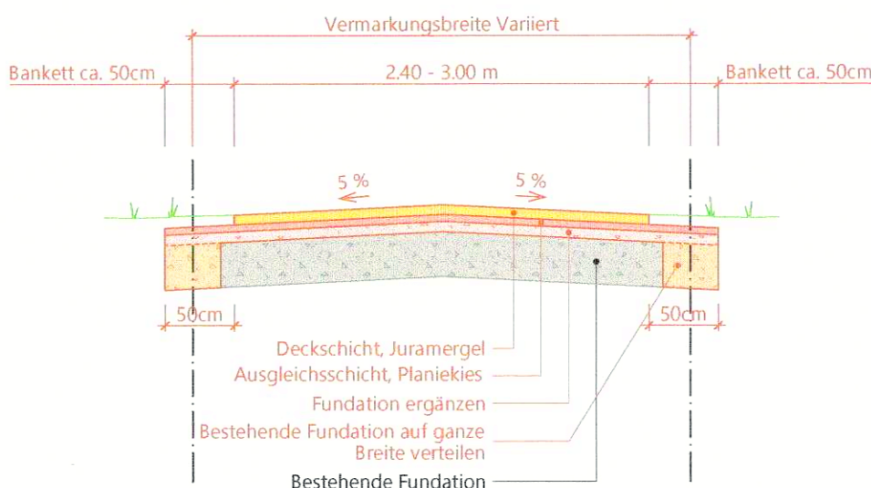
Normalprofil 1:50 Mergelweg: Fundationsergänzung & Verbreiterung Deckschicht
