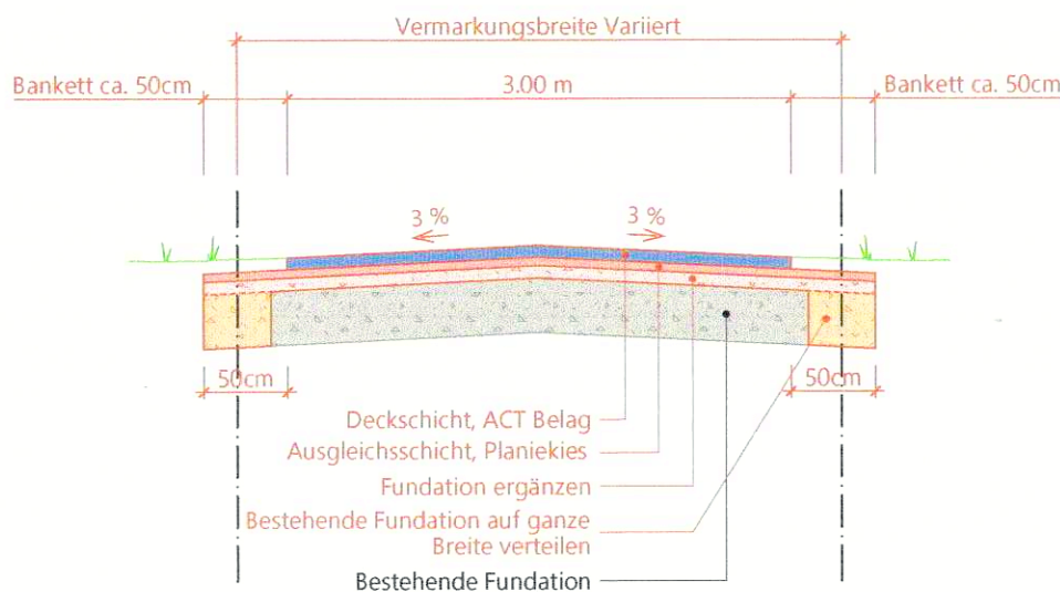
Normalprofil 1:50 ACT: Fundationsergänzung & Erneuerung Deckschicht
