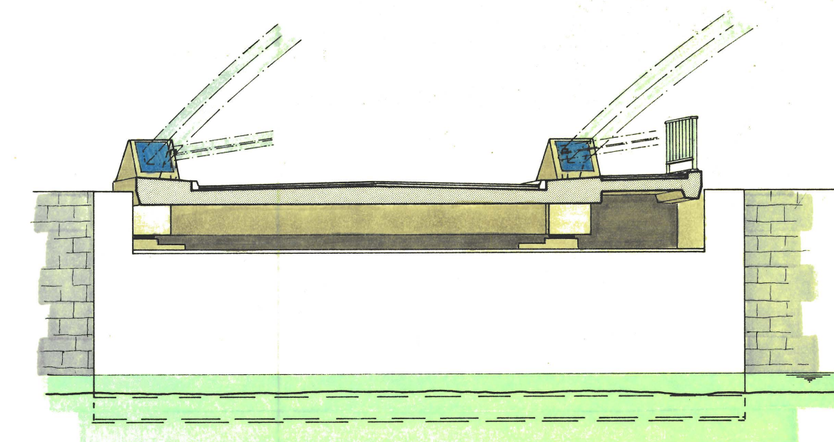
SCHNITT B-B 1:100
