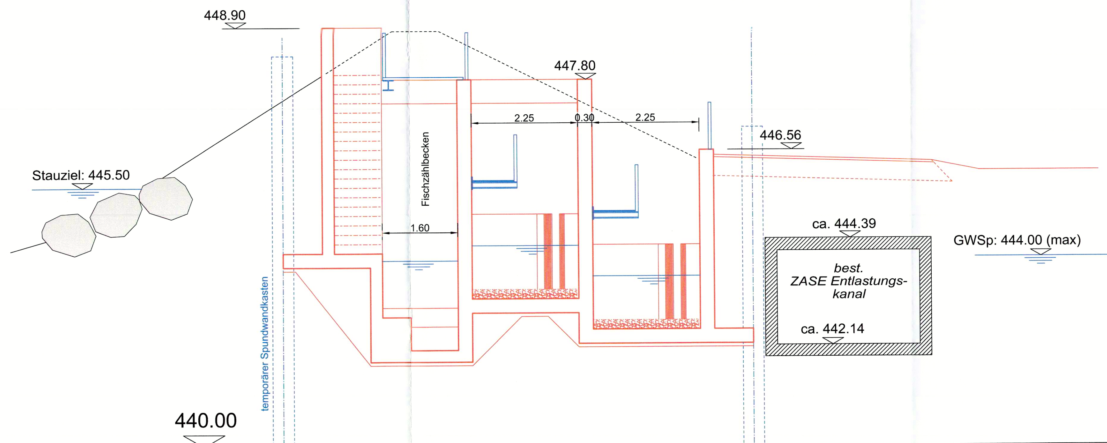
Schnitt C - C, 1 : 50
