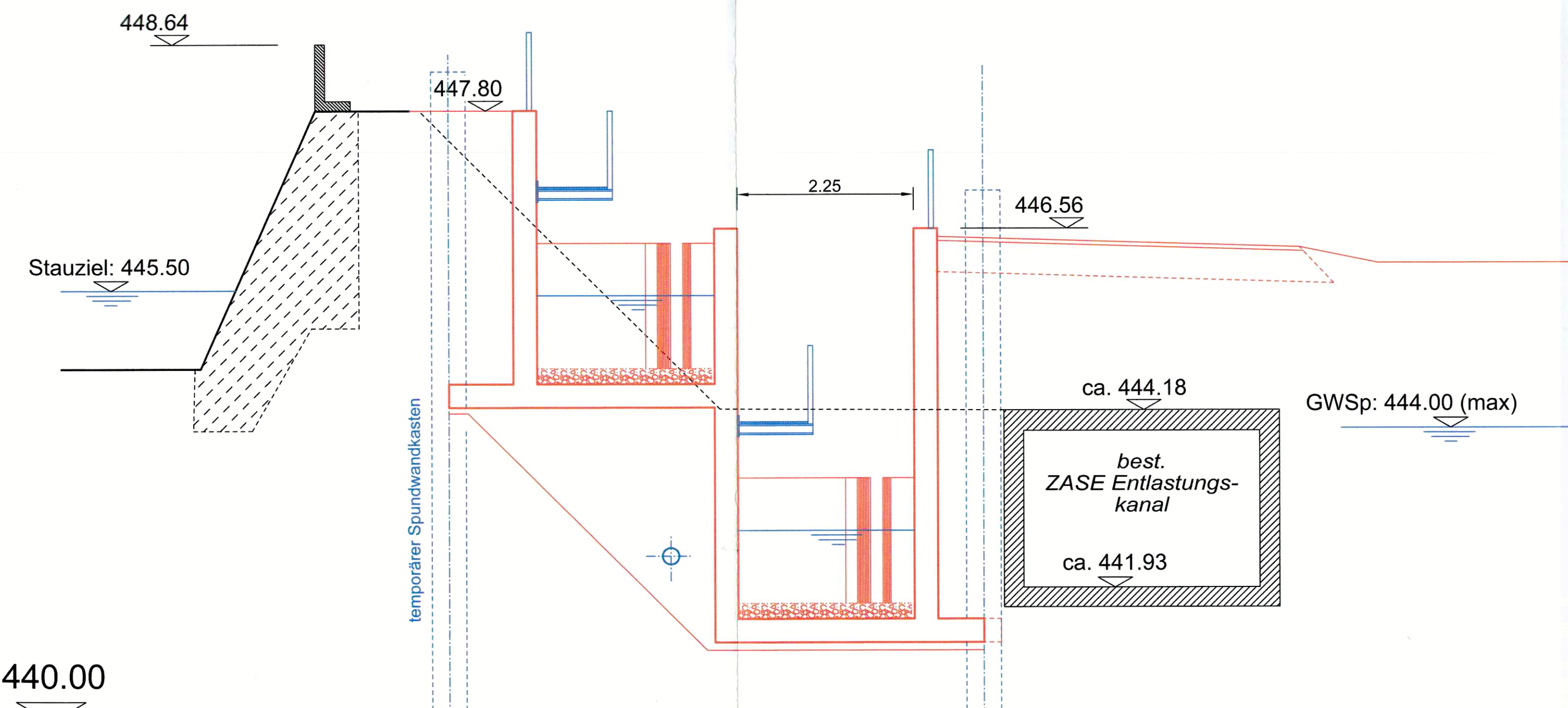
Schnitt B - B, 1 : 50
