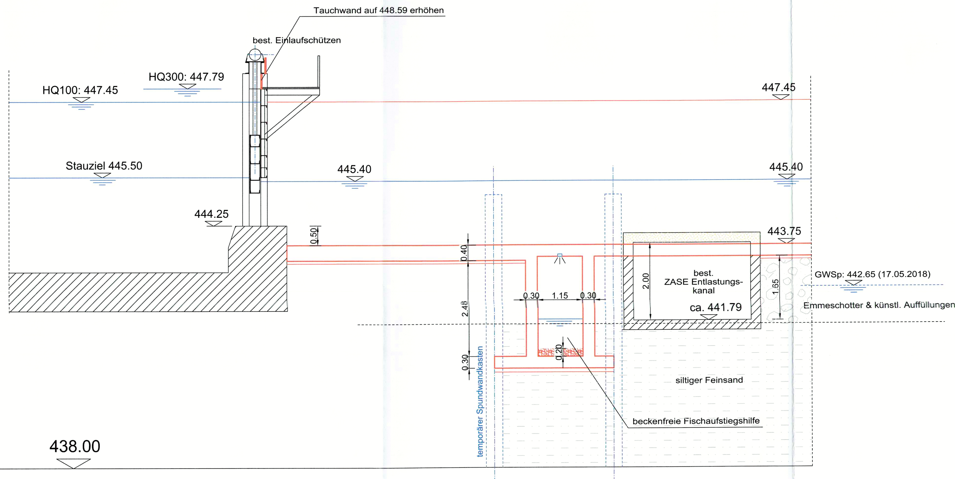
Schnitt A - A , 1 : 50
