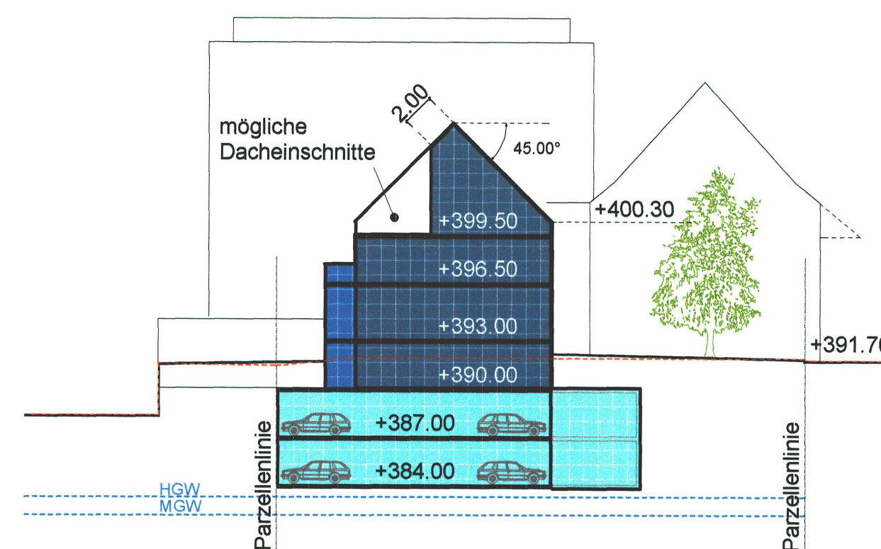
SCHNITT D-D' 1:333
