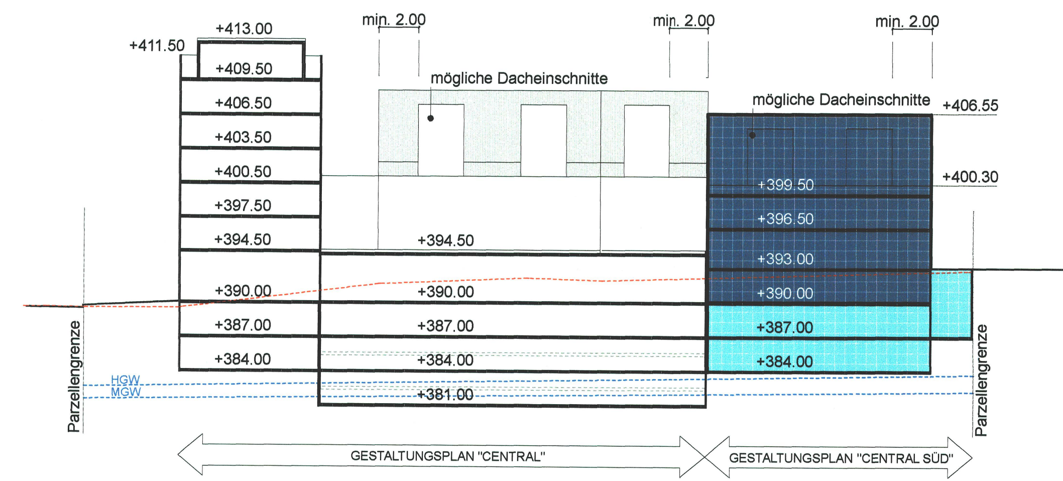
SCHNITT A'-A' 1:333
