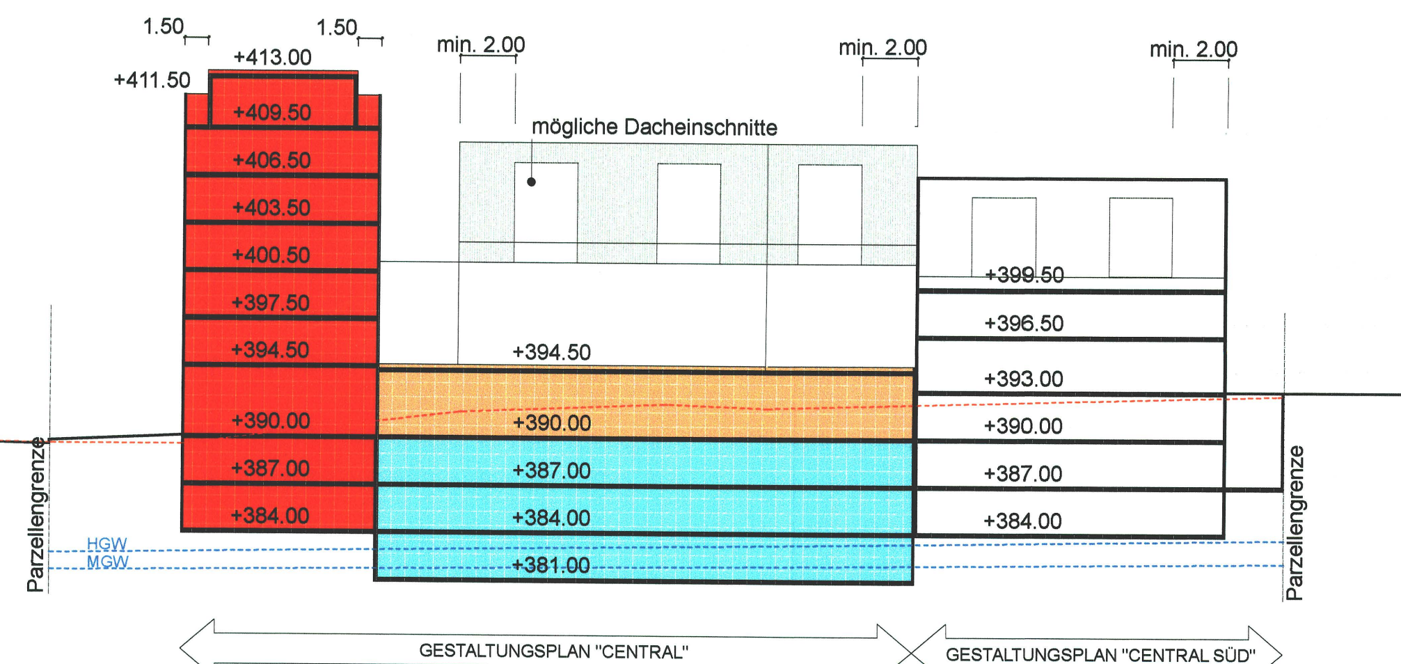
SCHNITT A-A 1:333
