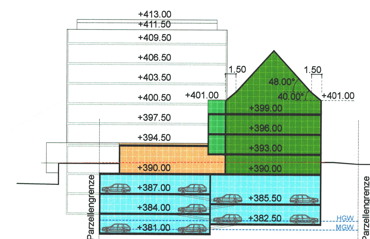
SCHNITT C-C 1:333
