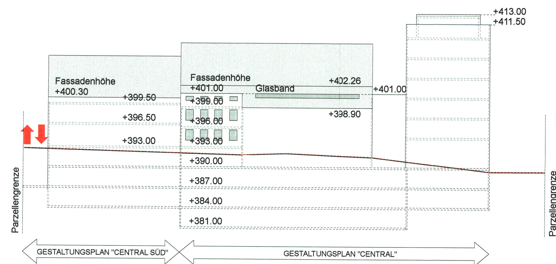
Ansicht B1 + B2 1:333
