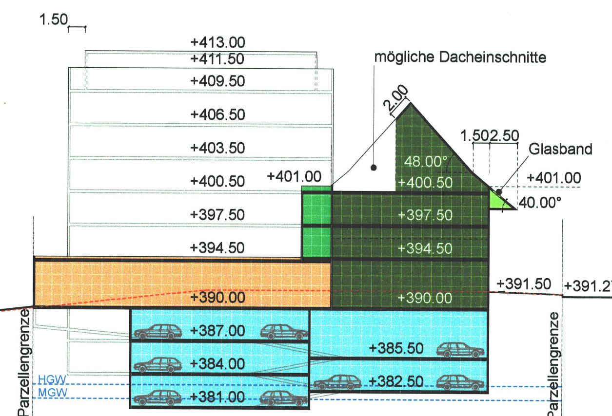
SCHNITT B-B 1:333
