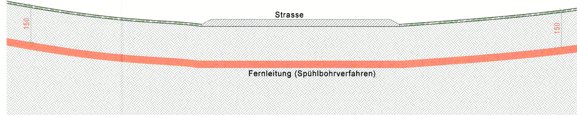
Strassenquerschnitt (Spühlbohrung)
