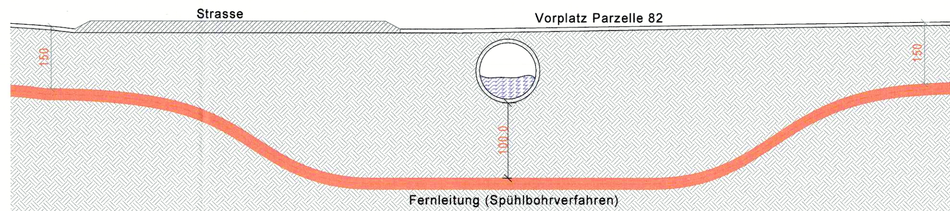
Strassenquerschnitt (Spühlbohrung)
