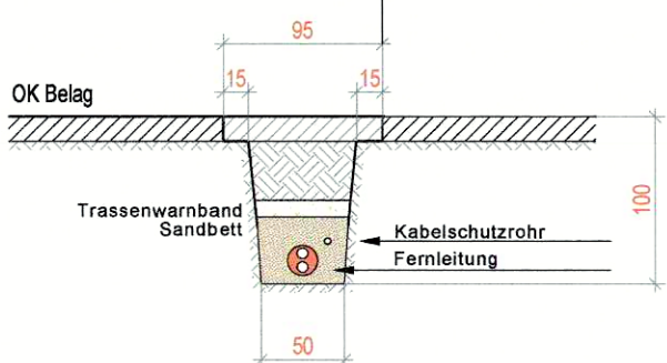
Grabenquerschnitt (Belag)
