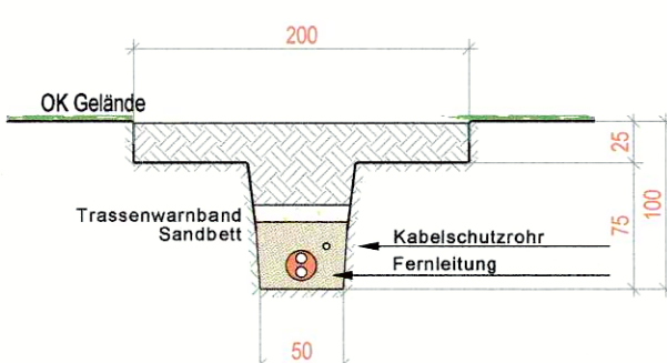
Grabenquerschnitt (Grünfläche)
