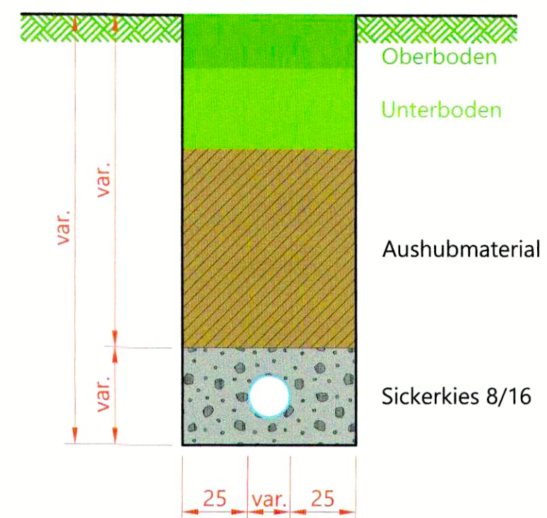
Querschnitt 1:20 Detail Sammelleitung
