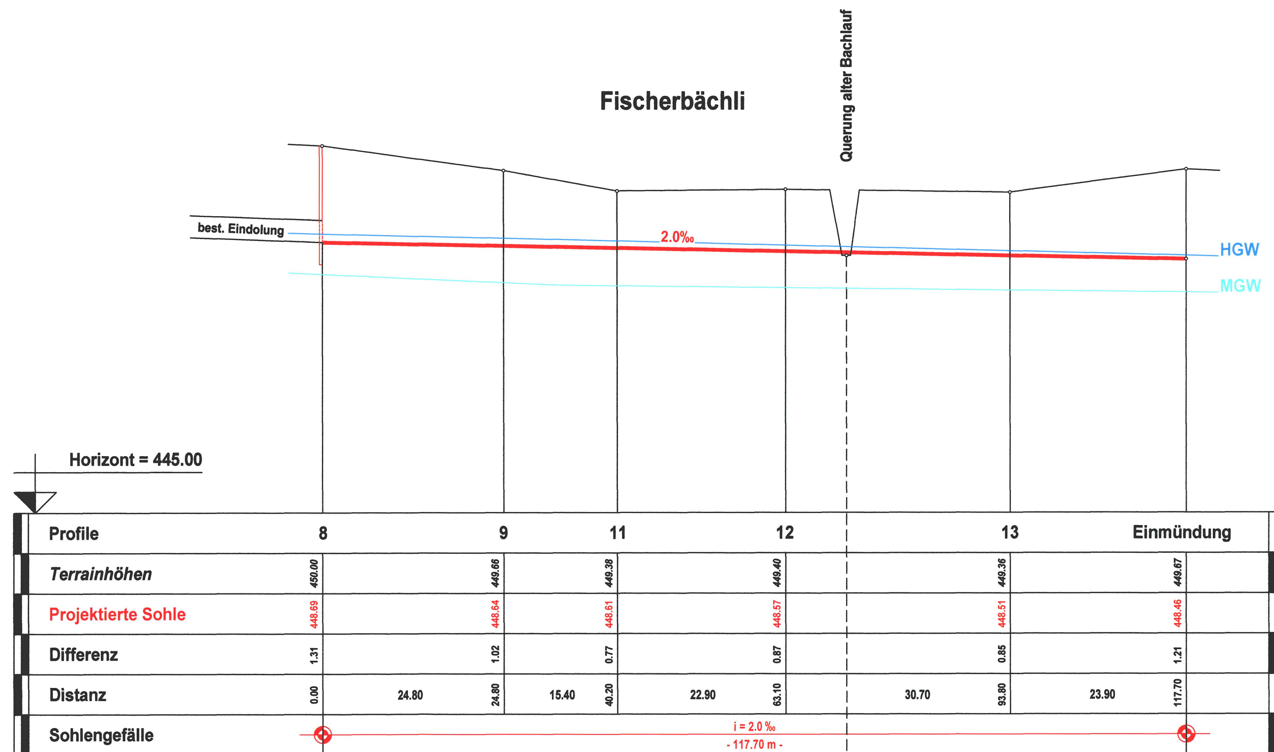
Längenprofil 1 : 500/50
