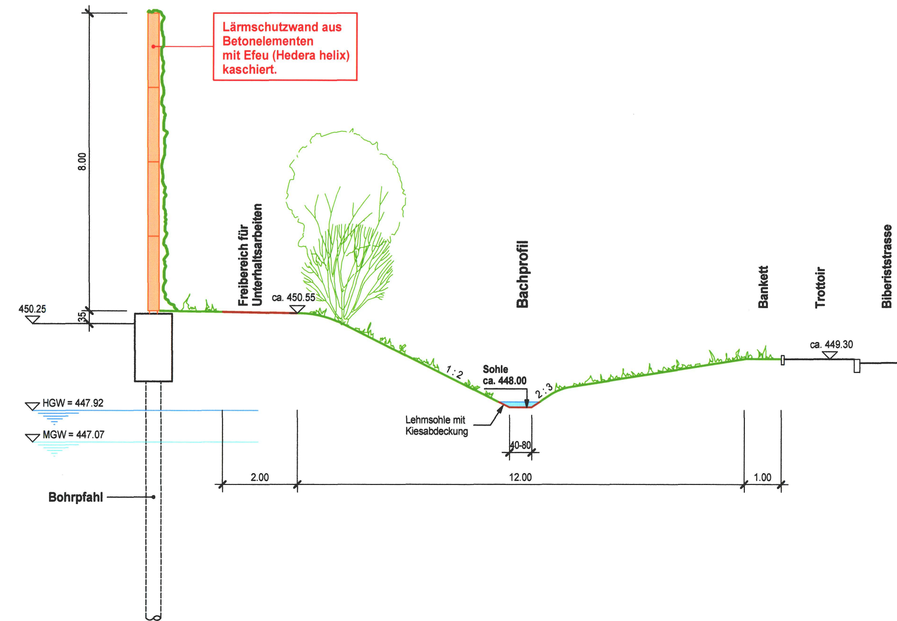
Normalprofil 1 : 100
