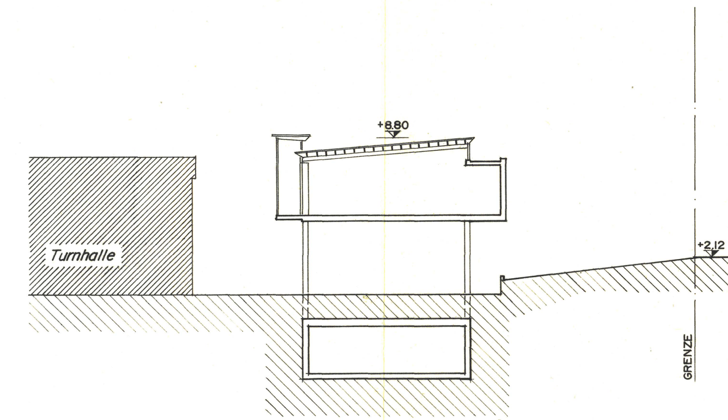
SCHNITT A-A
