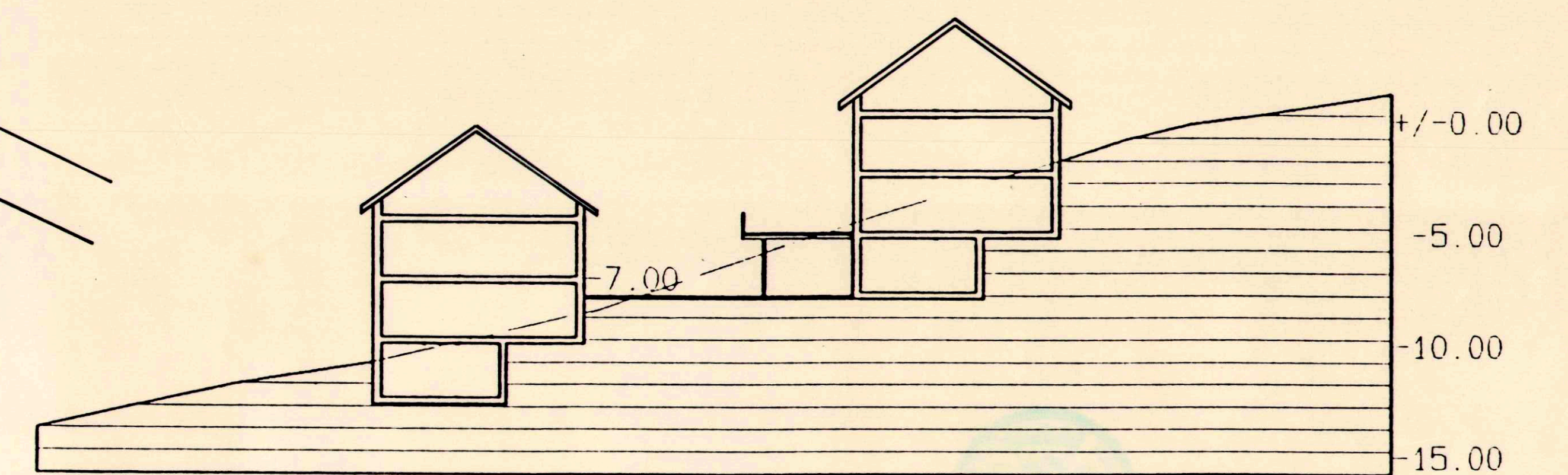
Terrainschnitt B-B
