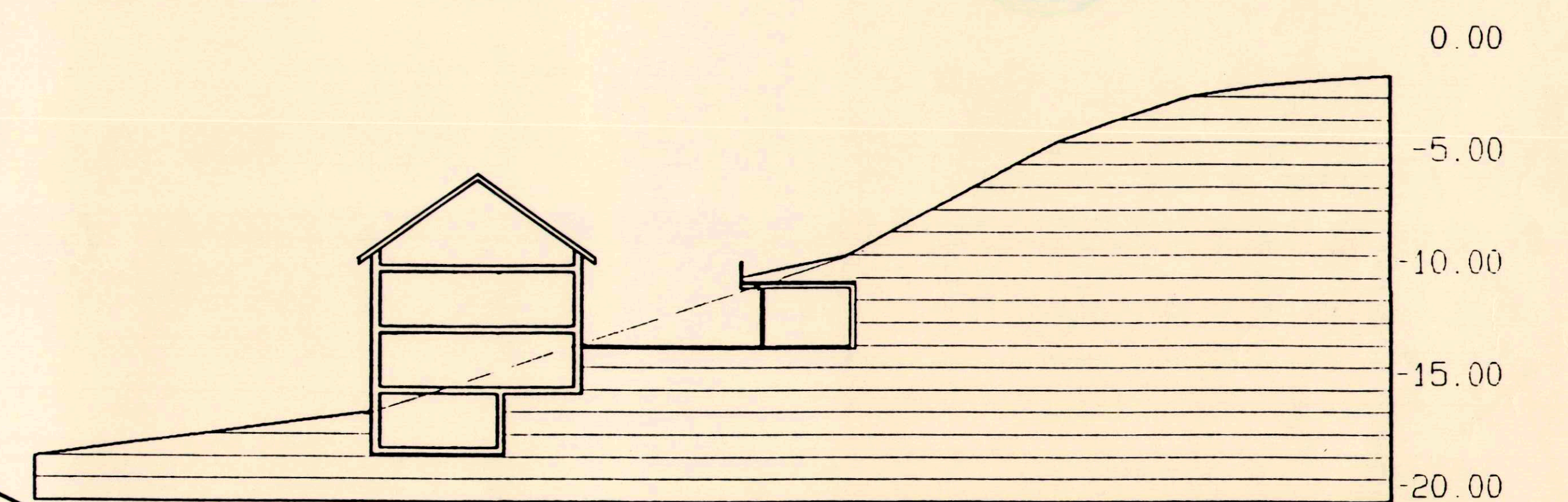
Terrainschnitt C-C
