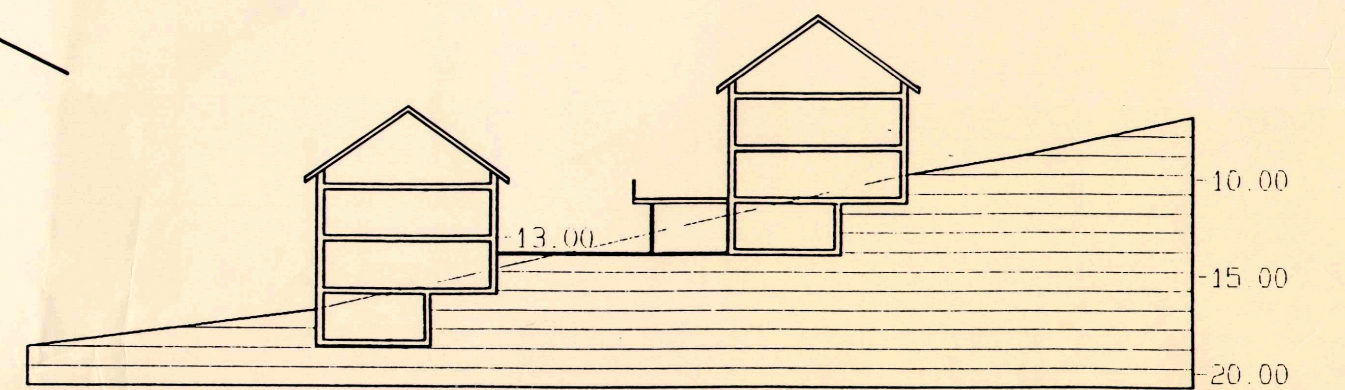
Terrainschnitt D-D
