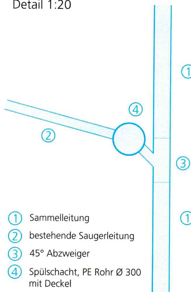
Anschluss Drainageleitung Detail 1:20
