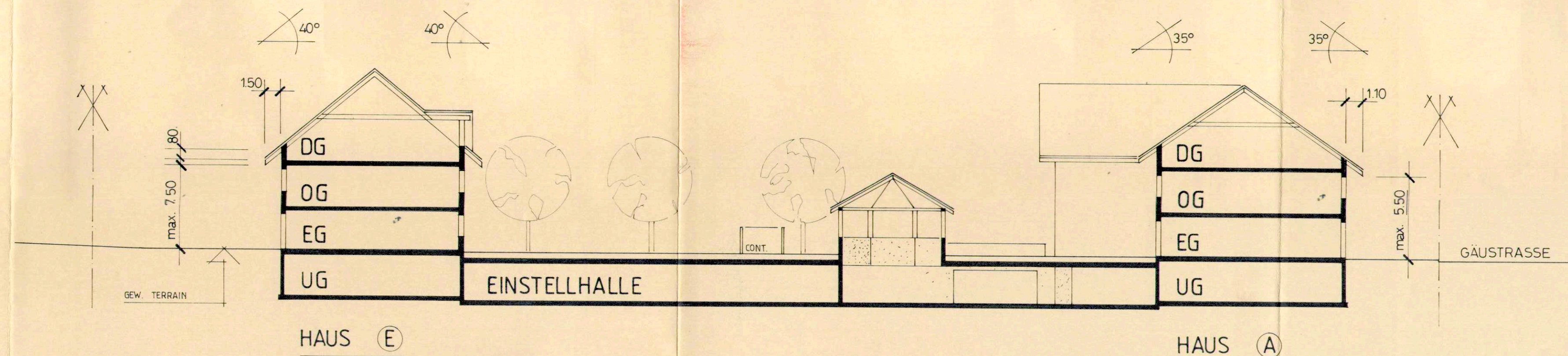
QUERSCHNITT A - A 1:200
