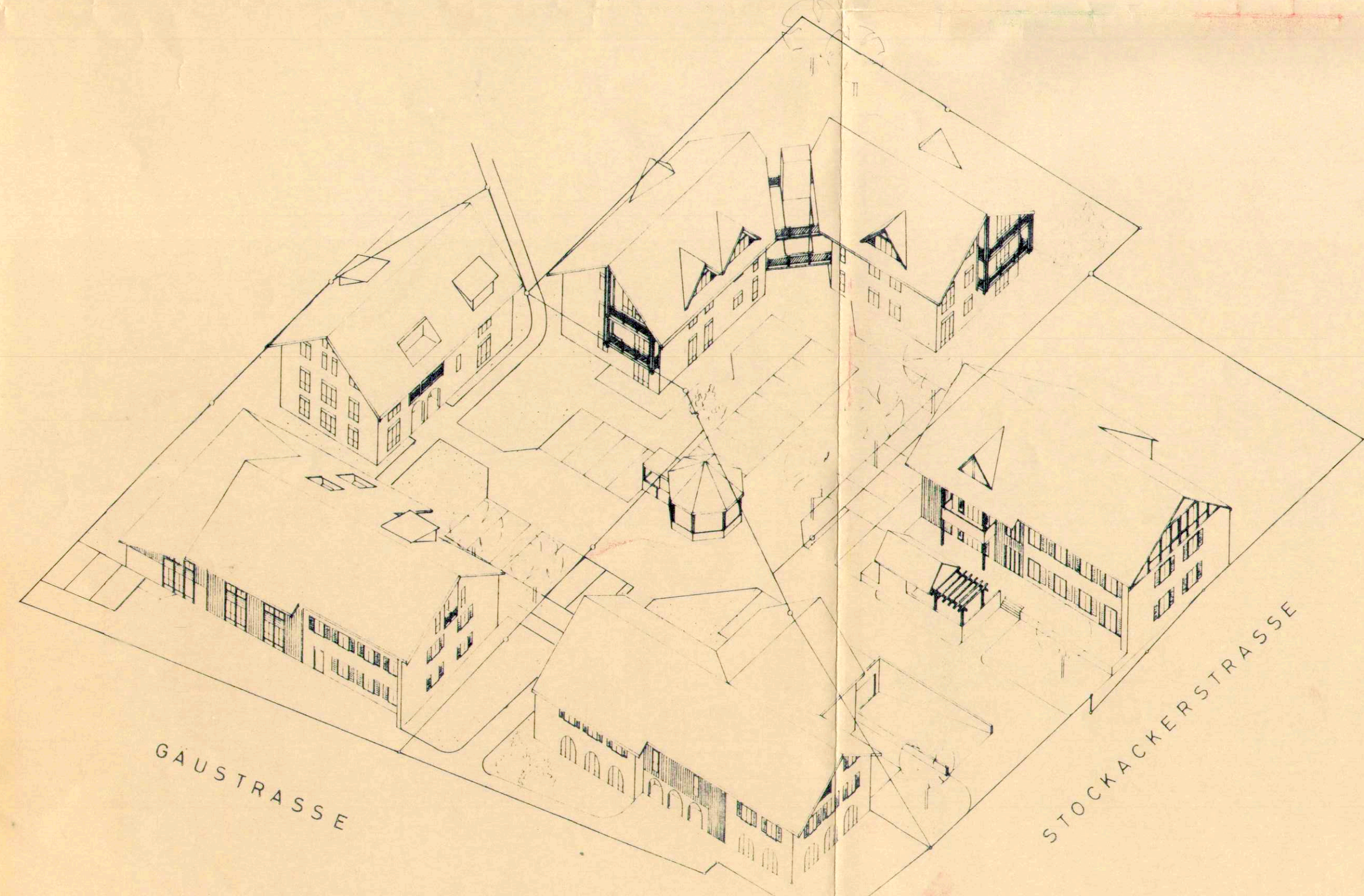
ISOMETRIE 1:400
