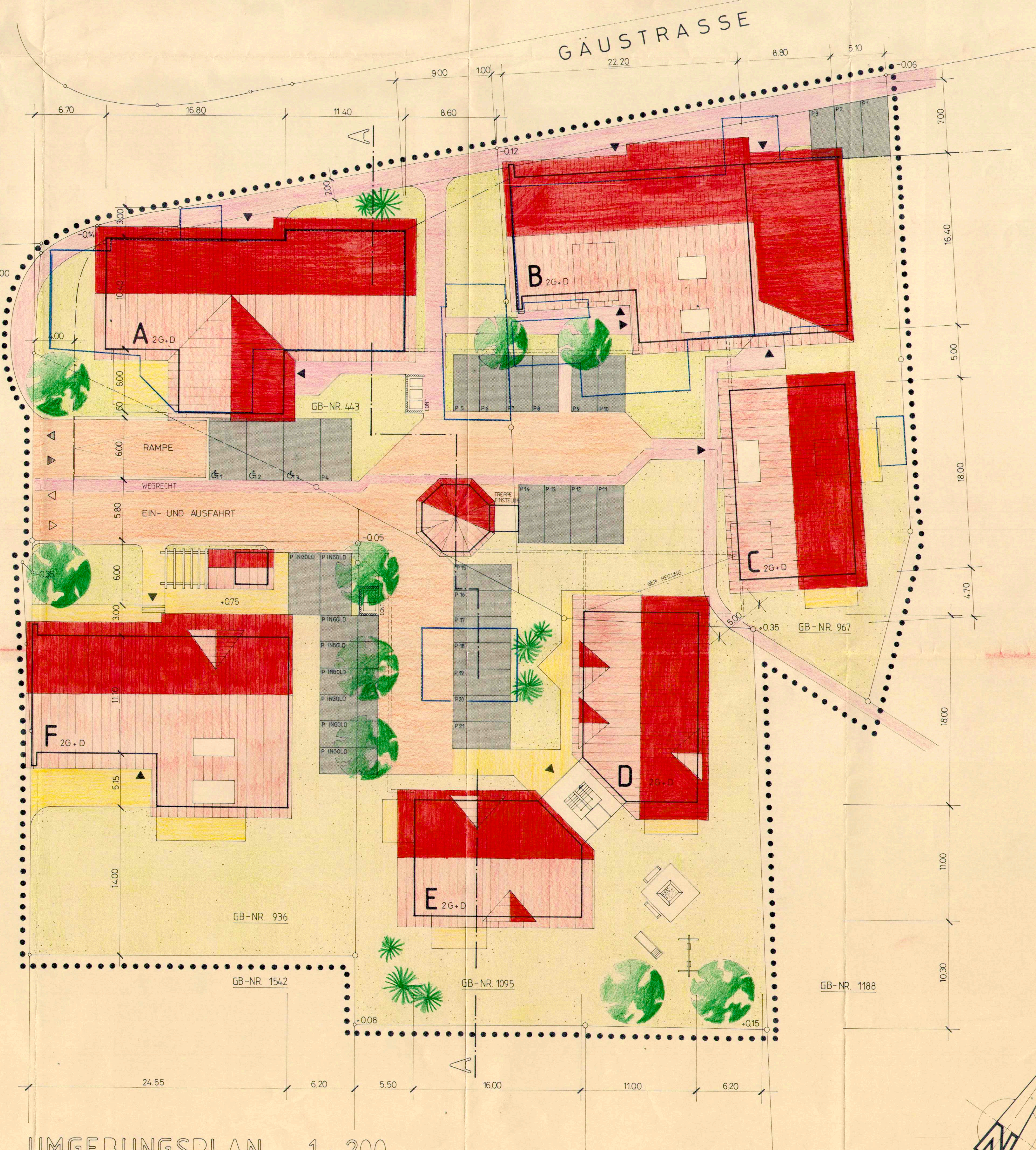
UMGEBUNGSPLAN 1:200
