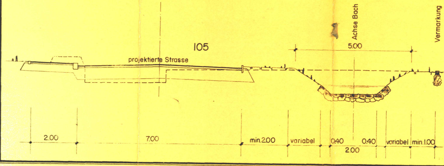
Korrektur Maccaronibach Typisches Querprofil 1:100
