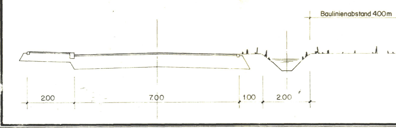
Korrektur Gehrengaben Querprofil 1:100
