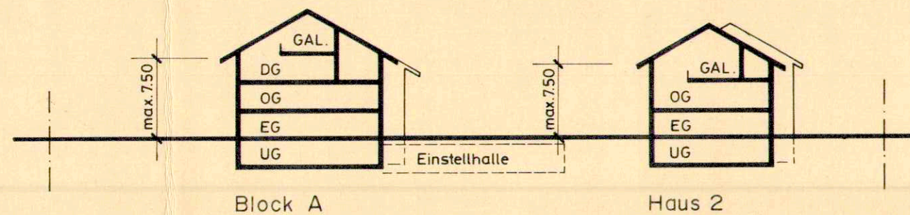
Schemaschnitt X-X
