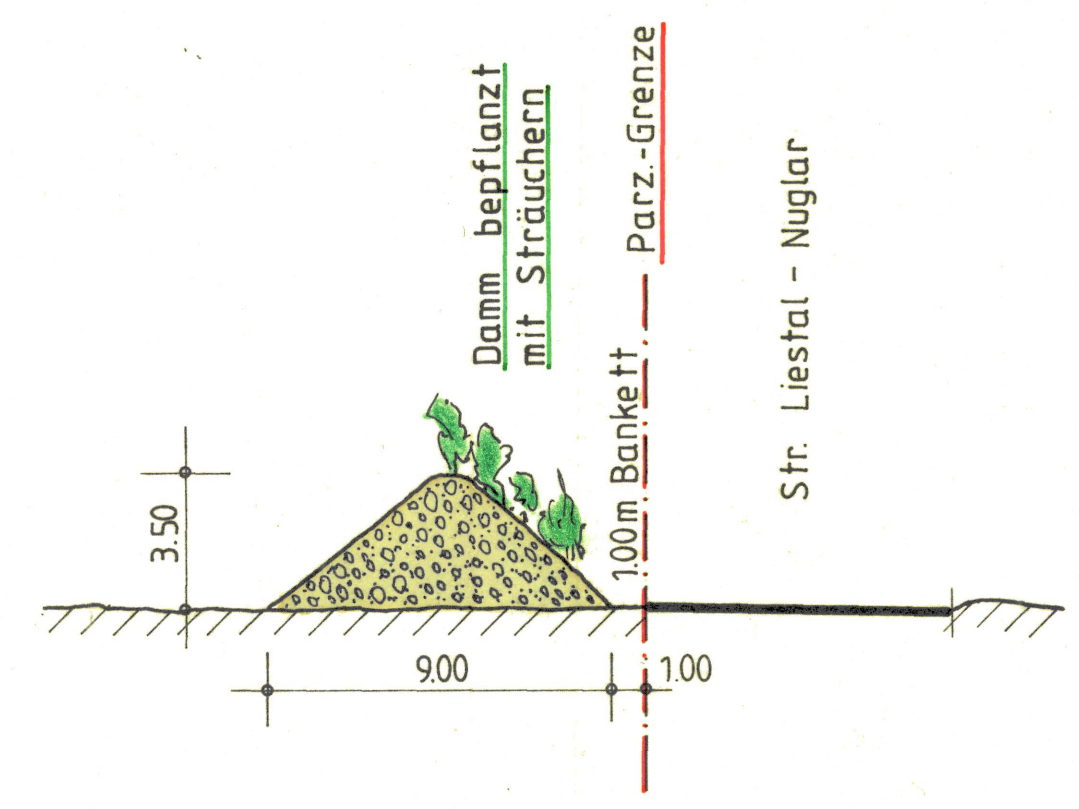
SCHNITT B-B, 1 : 200
