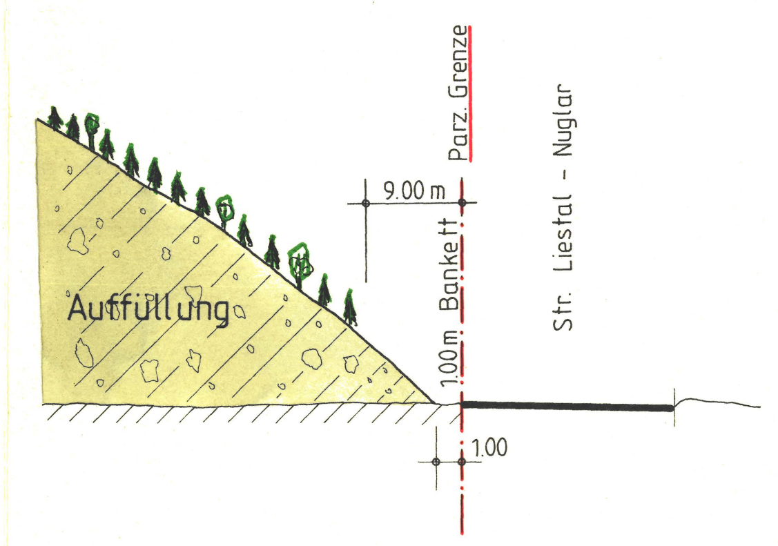
SCHNITT B-B, 1:200
