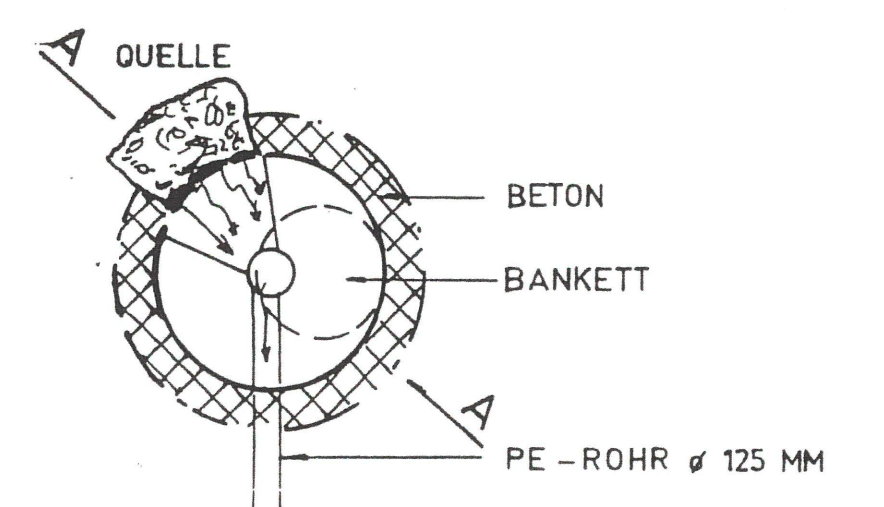
GRUNDRISS M. 1:50
