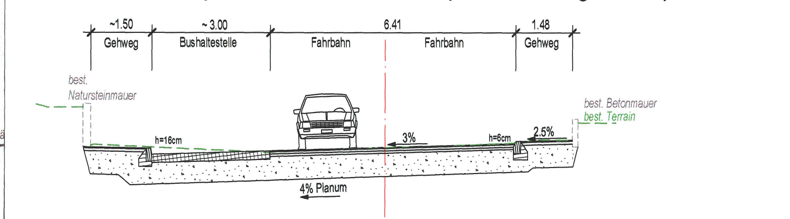
Schemaquerschnitt B-B 1:100 (Orientierungsinhalt)
