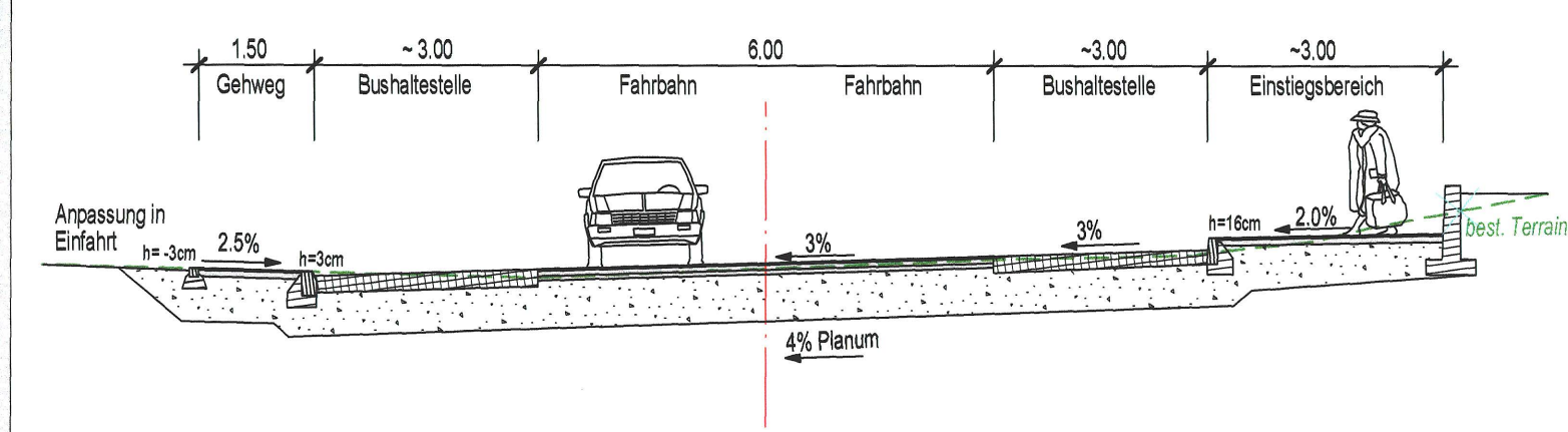
Schemaquerschnitt A-A 1:100 (Orientierungsinhalt)
