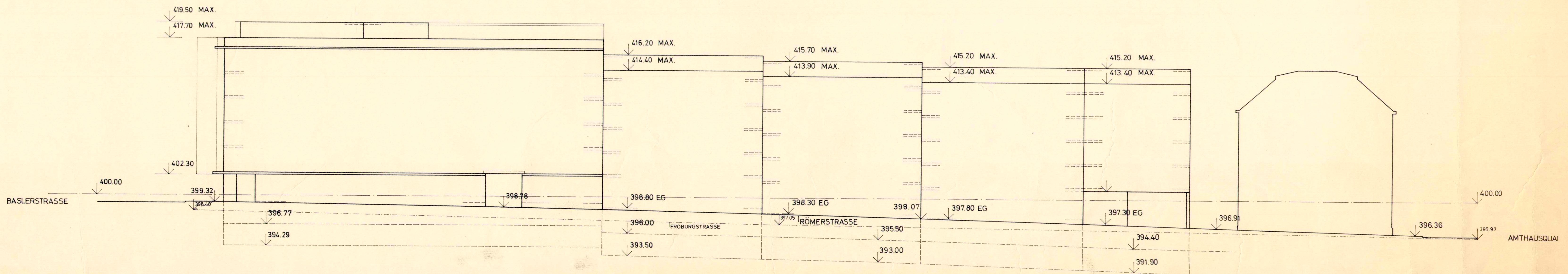
ANSICHT RÖMERSTRASSE
