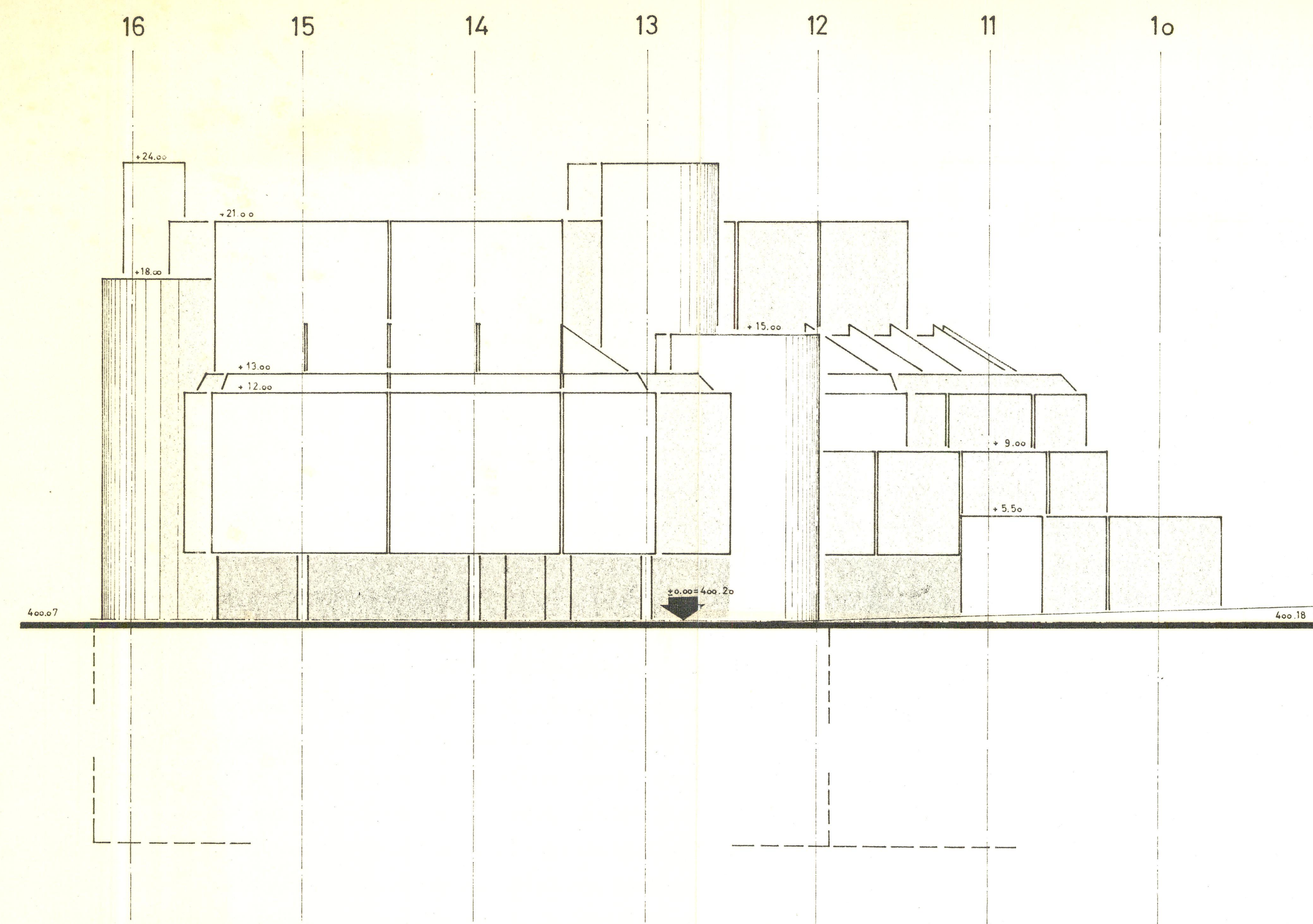
ANSICHT SOLOTHURNERSTRASSE
