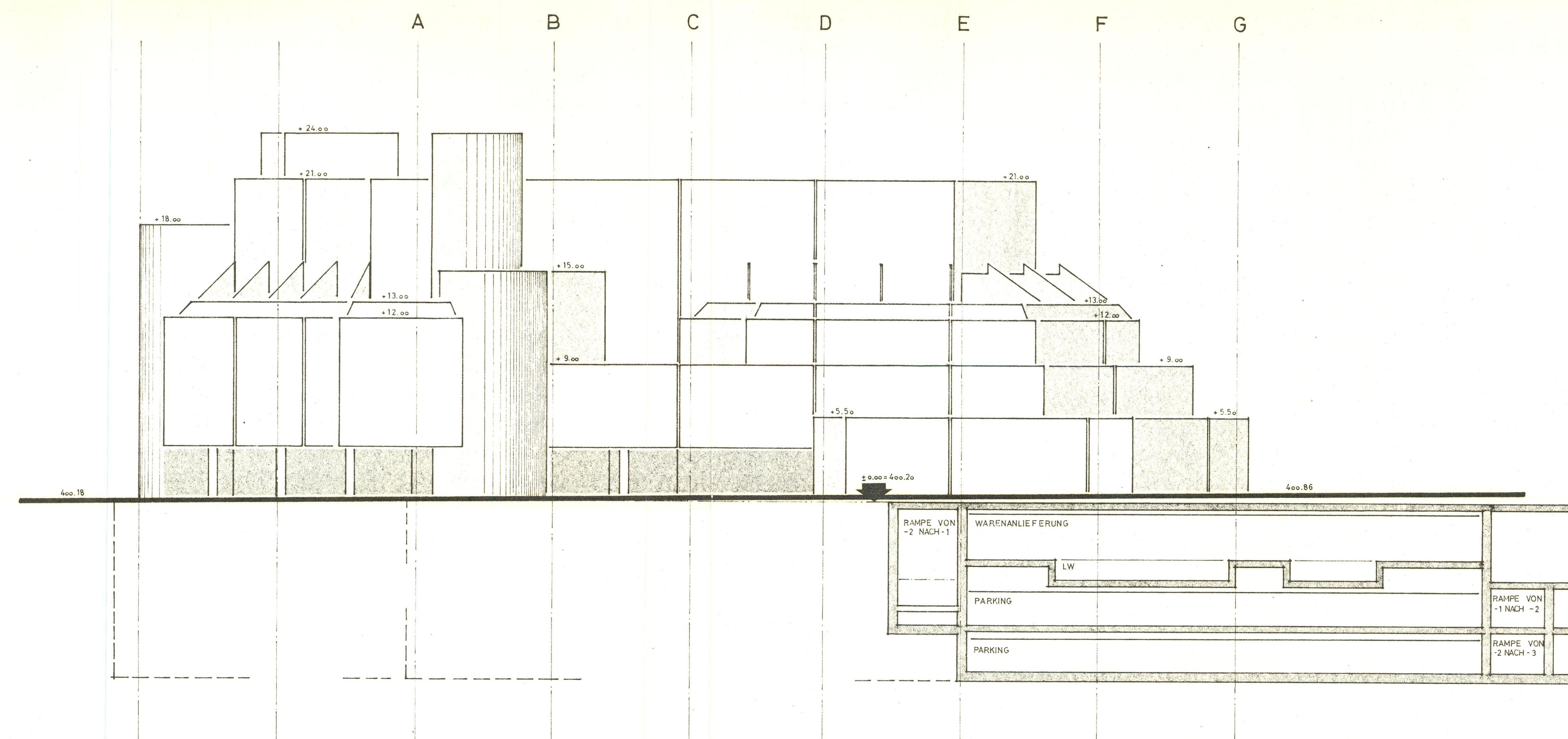
ANSICHT HAMMERALLEE
