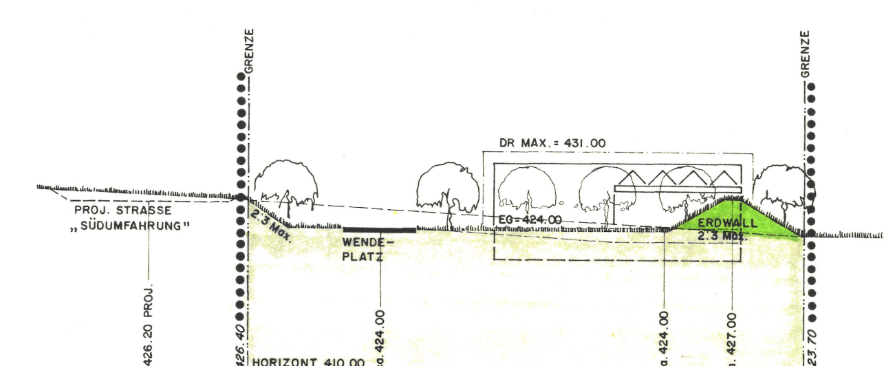
Nord-Ost Ansicht c-c
