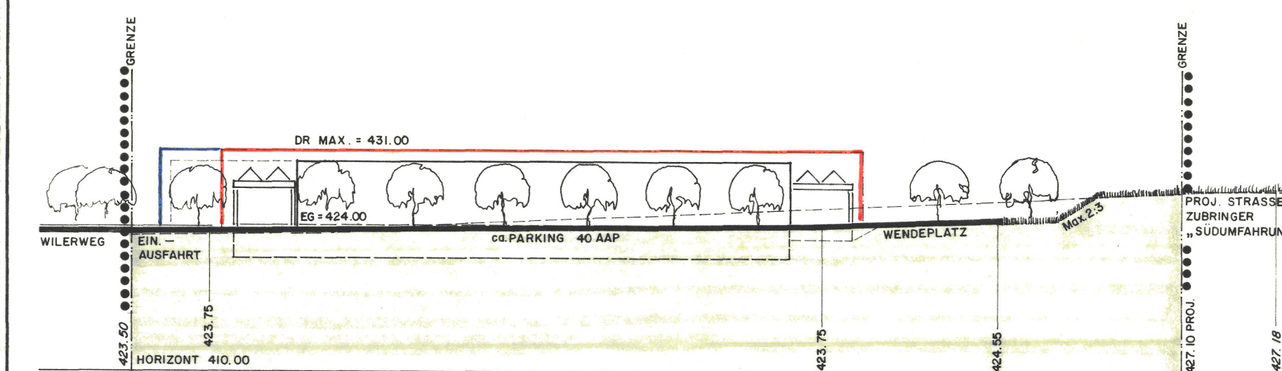
Süd-Ost Ansicht d-d
