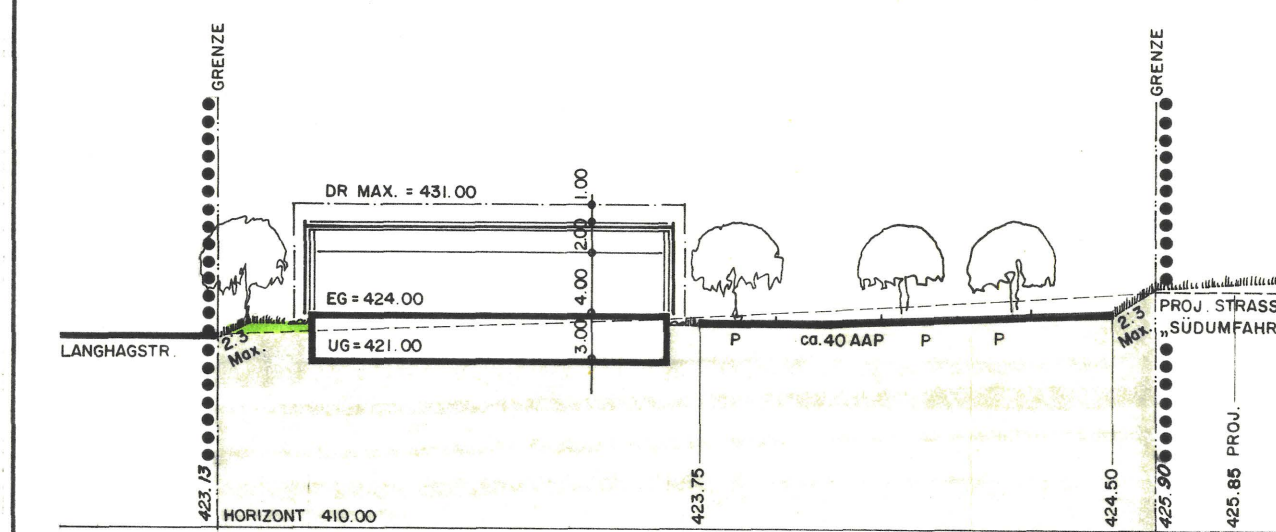
Schnitt a-a
