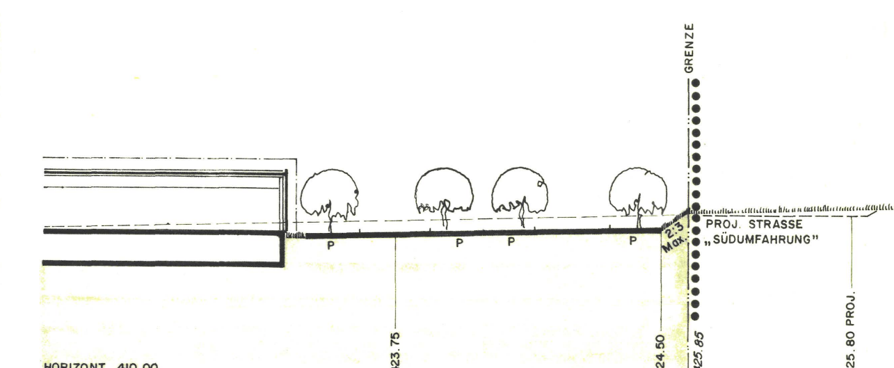
Schnitt h-h
