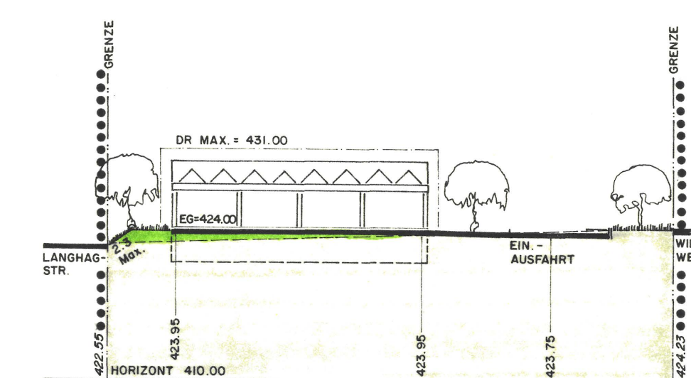
Süd-West Ansicht b-b
