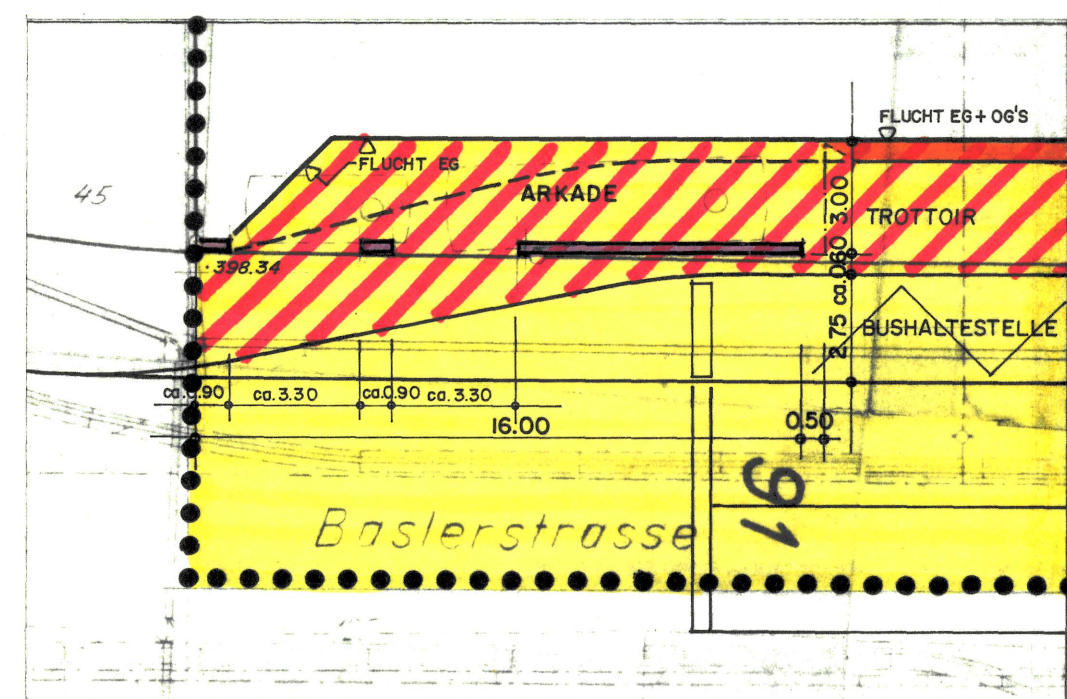
AUSSCHNITT ERDGESCHOSS BEREICH ARKADE M 1:200
