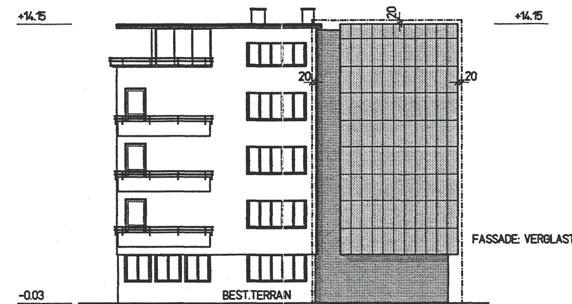
OSTFASSADE
