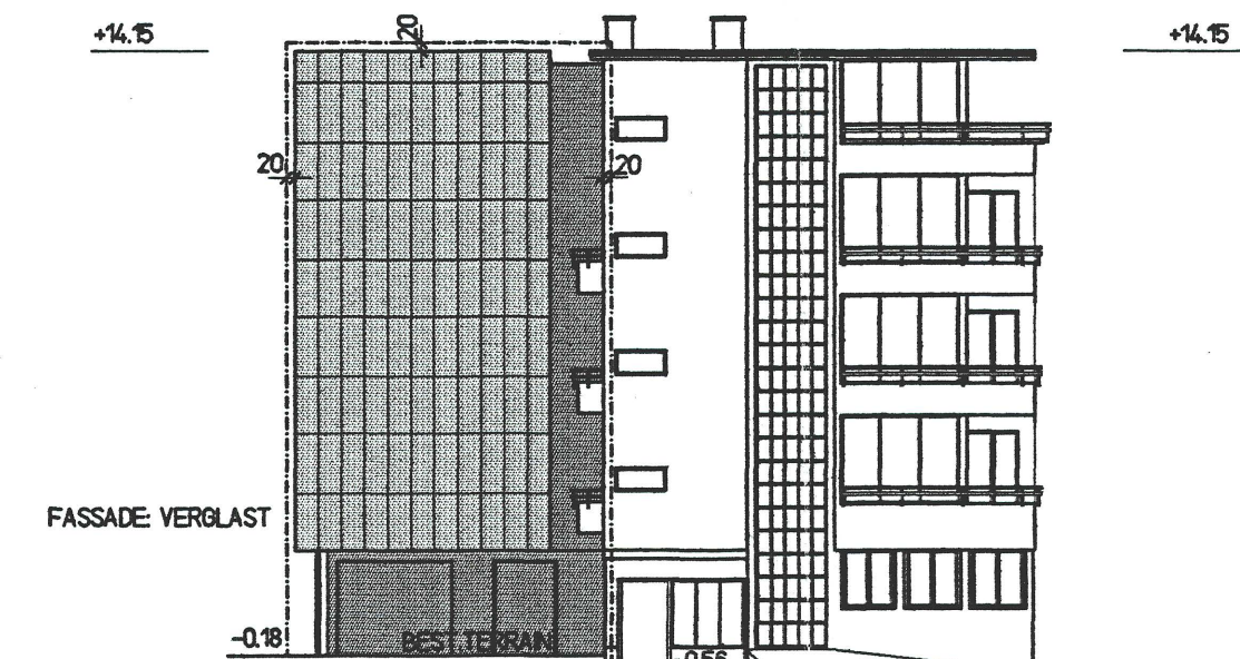
WESTFASSADE
