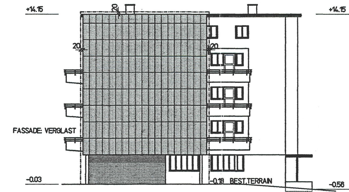
NORDFASSADE
