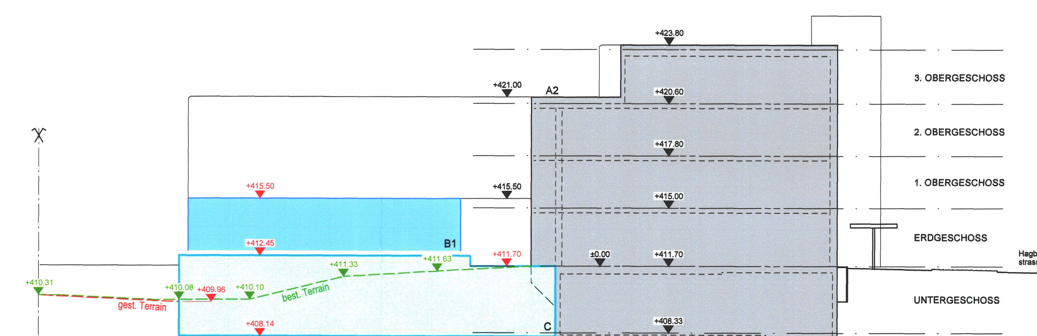
SCHNITT 2
