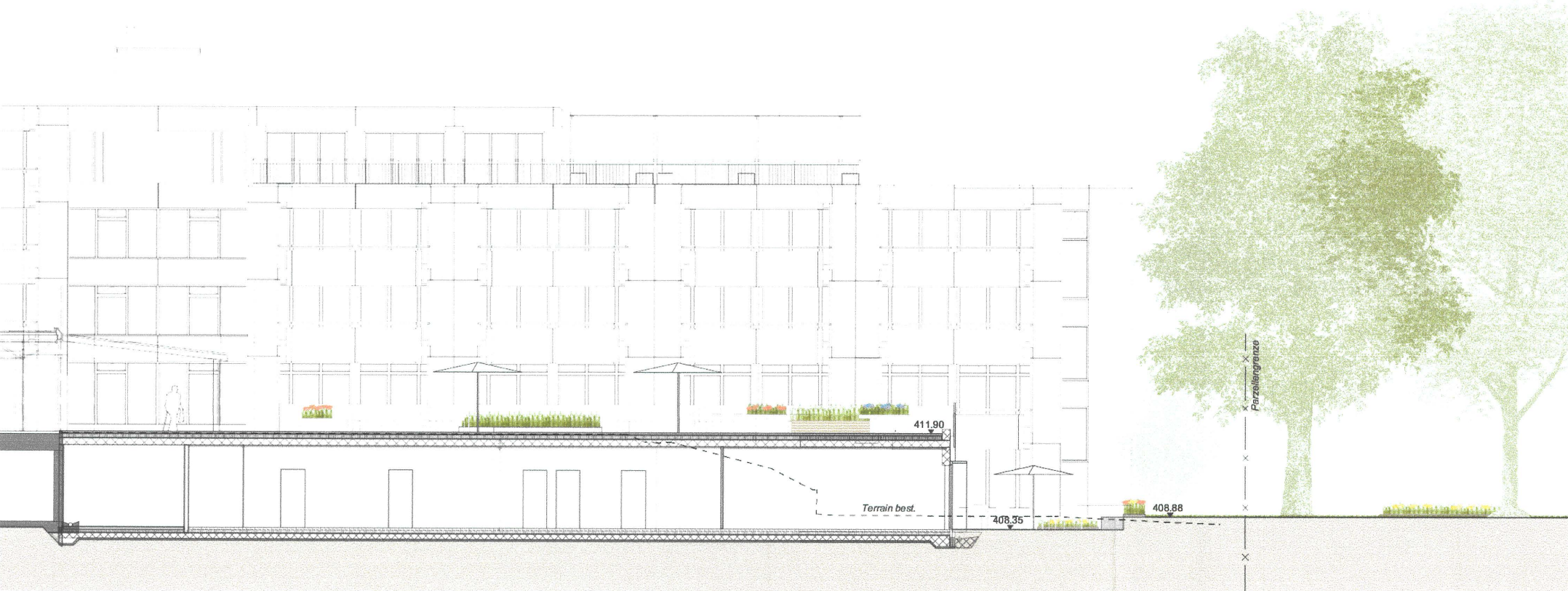
Schnitt A-A 1:200
