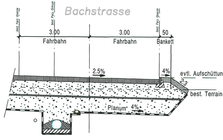
Schemaquerschnitt Bachstrasse (Orientierungsinhalt)
