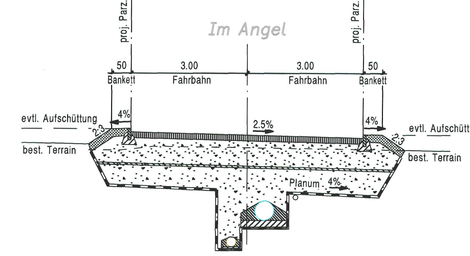
Schemaquerschnitt Im Angel (Orientierungsinhalt)
