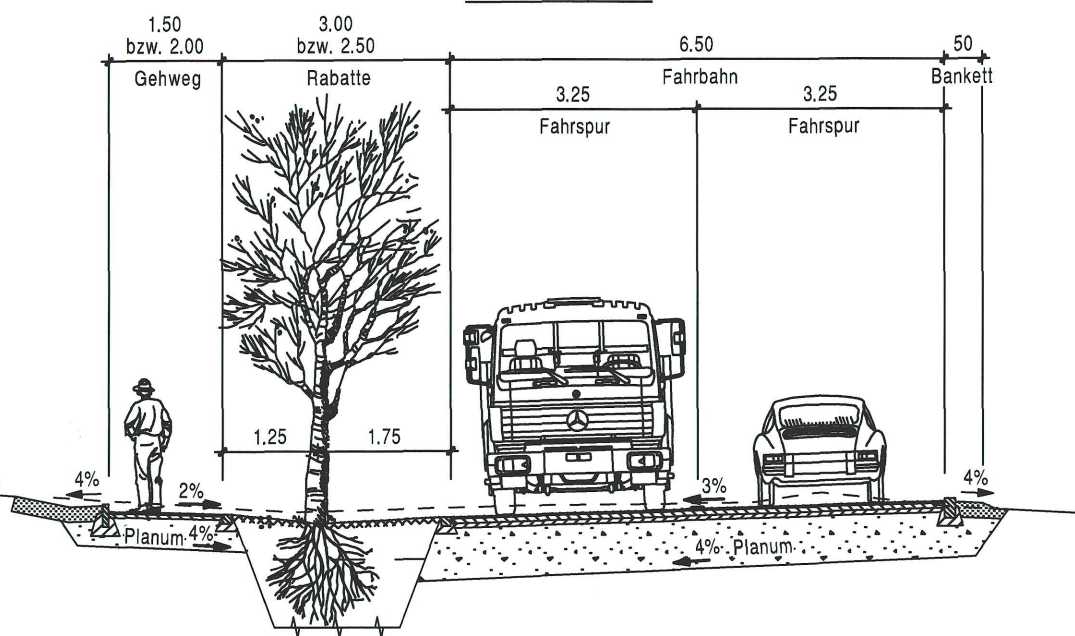
Schemaquerschnitt Grellingerstrasse (Orientierungsinhalt)
