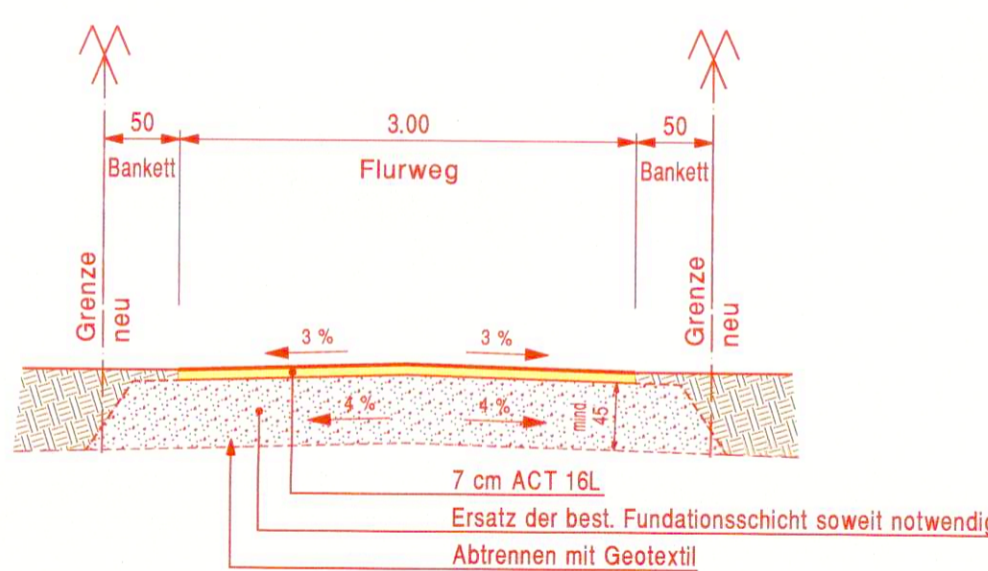
Normalprofil 1:50
