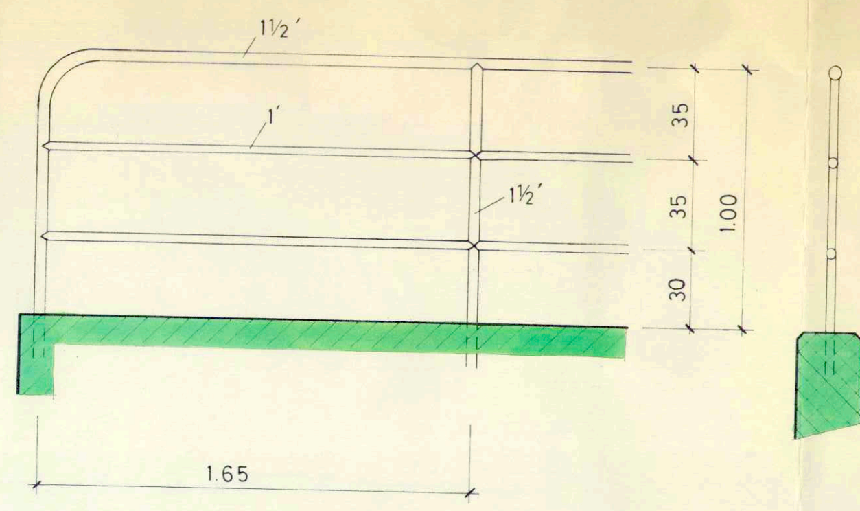
Rohrgeländer aus 1 1/2'+1'-Rohren verzinkt
