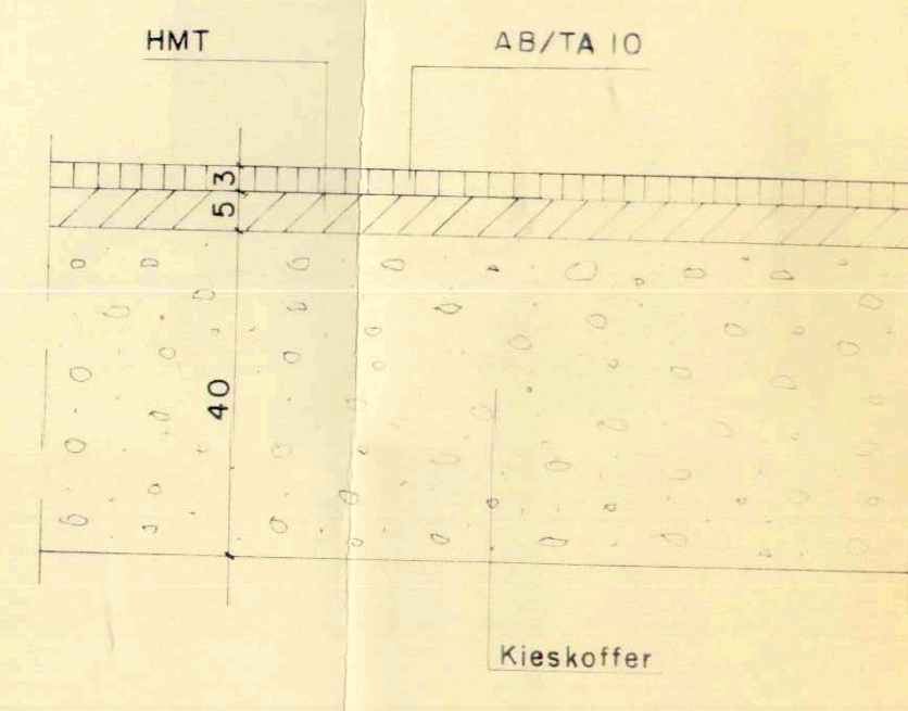
Gehwege Oberbau 1:10
