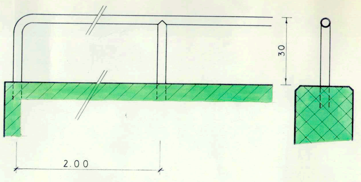
Rohrgeländer aus 1 1/2'-Rohren verzinkt
