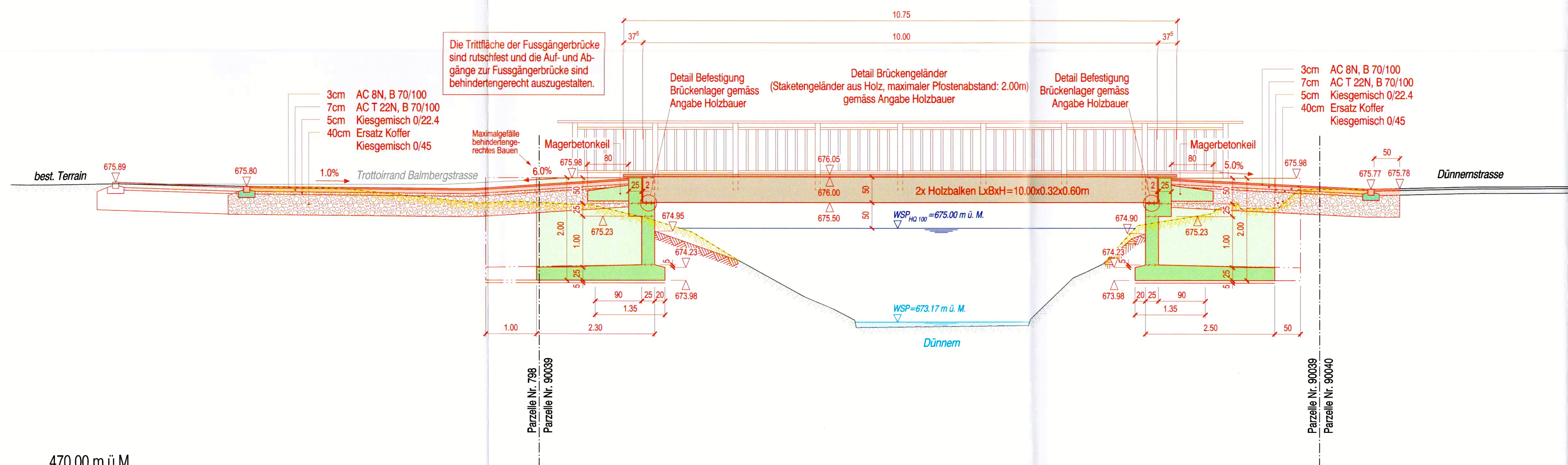
Schnitt A-A 1:50
