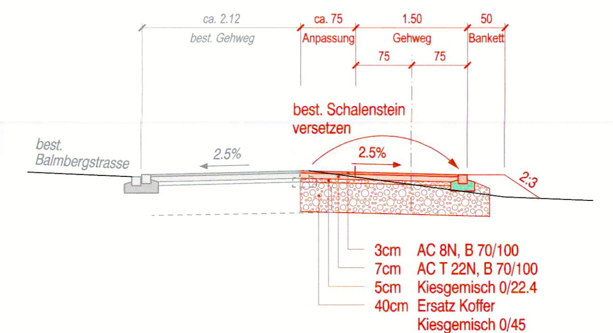
Querprofil 1:50
