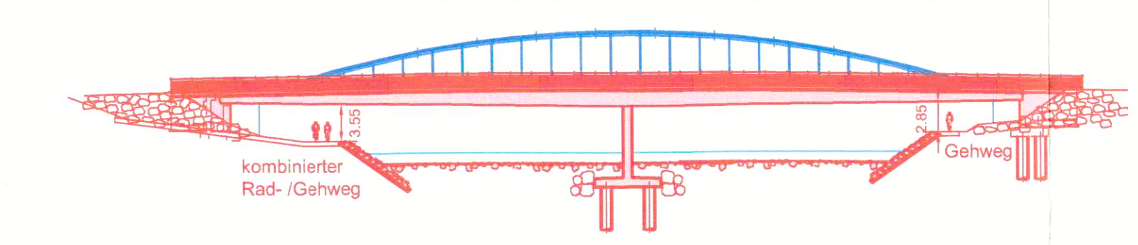
Ansicht Oberwasser 1:500
