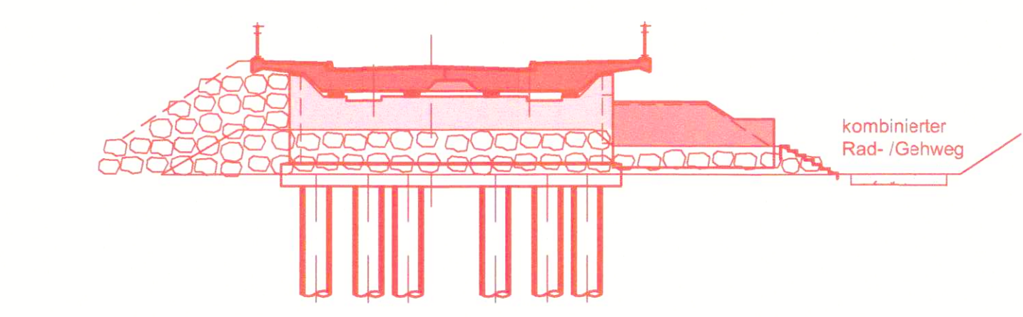
Ansicht Widerlager Seite Luterbach 1:200
