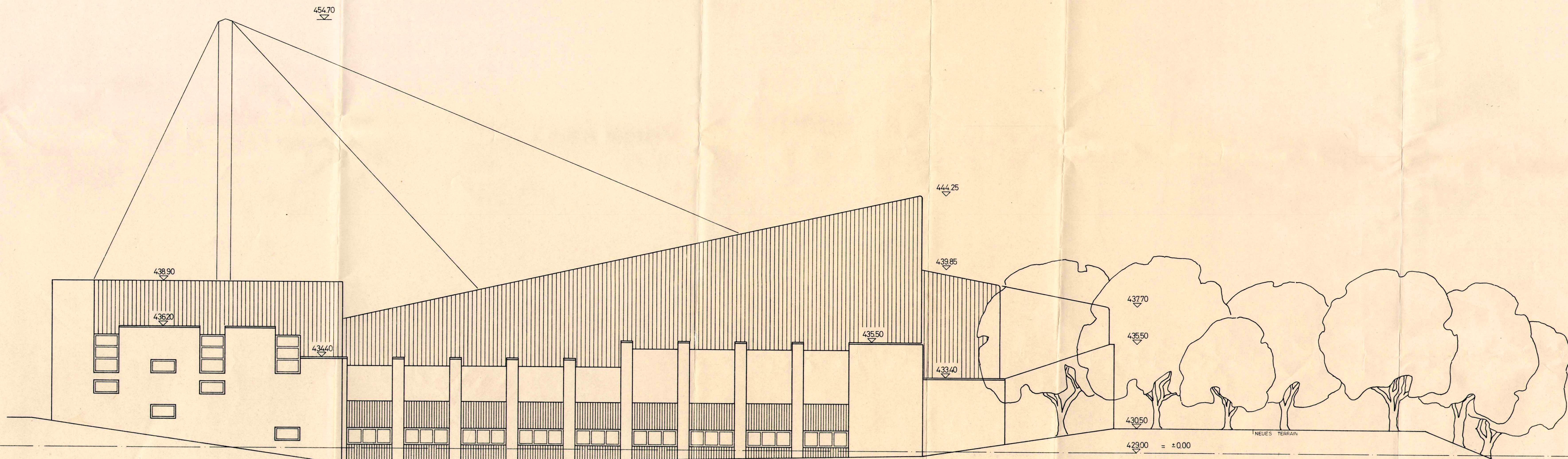
OSTANSICHT
