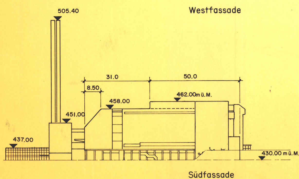
Südfassade
